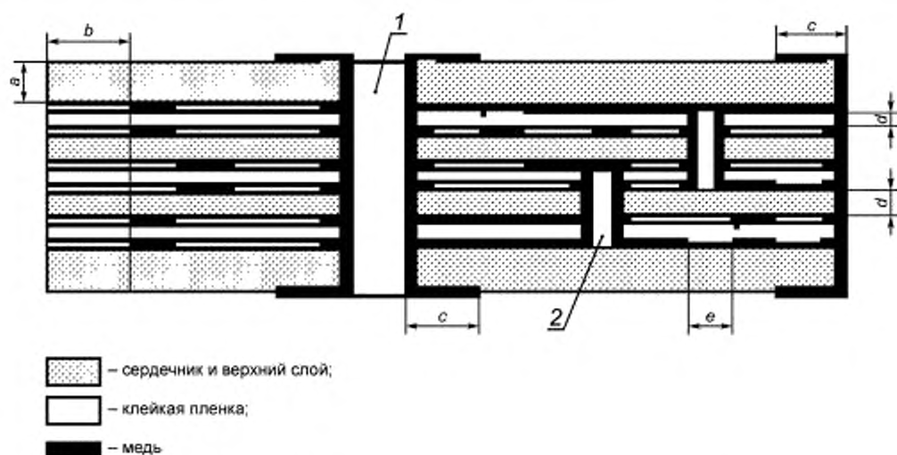
Рисунок 4 — Минимальные расстояния для многослойных печатных монтажных плат
