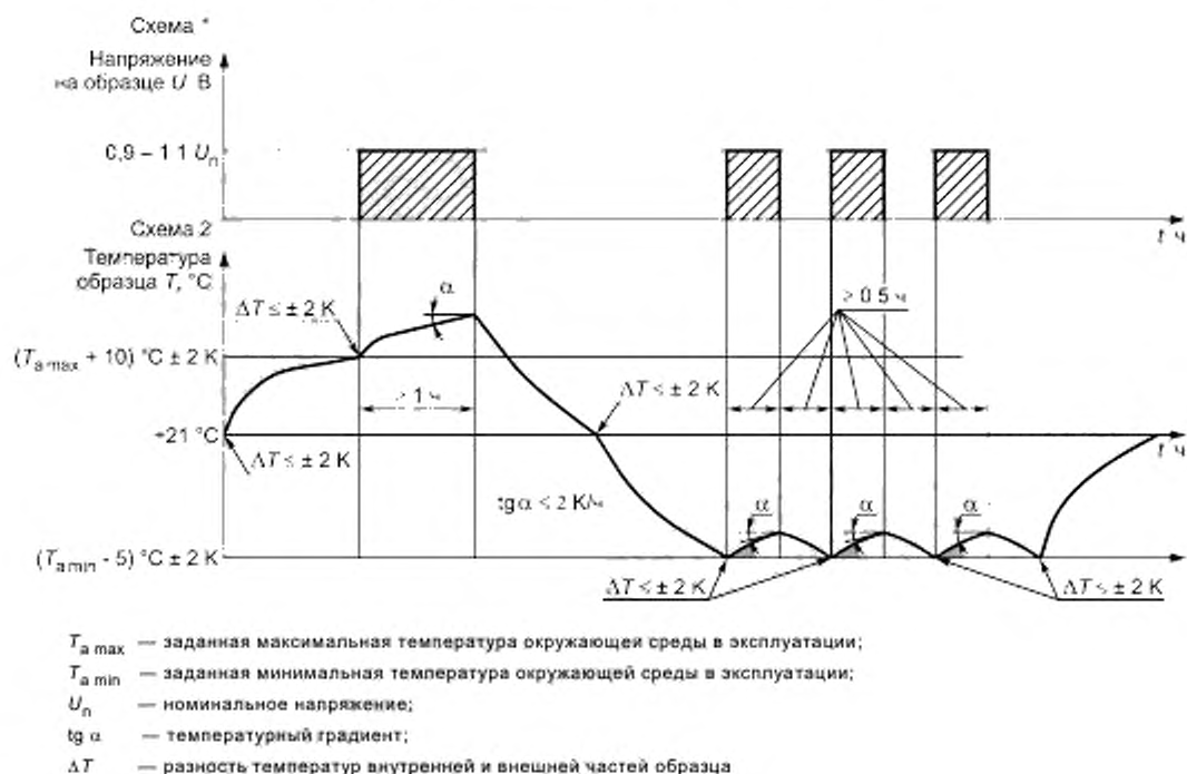
Рисунок С.1 — Методика проведения теплового циклического испытания
