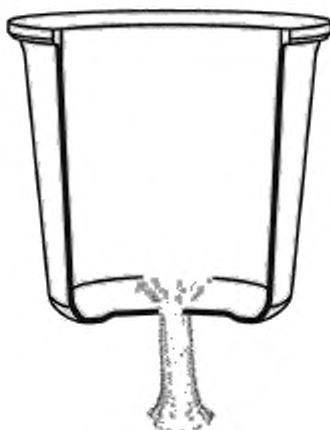
Рисунок 1 — Пример испытательного сосуда с фитилем из стекловолокна
