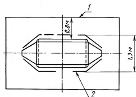
Схема расположения открытой Т-камеры в экранированном помещении
