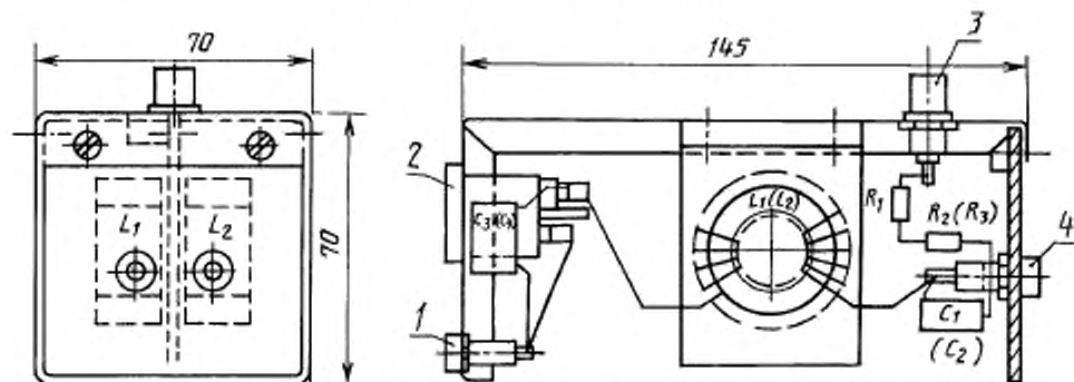
Блок связи типа М. Сборочный чертеж
