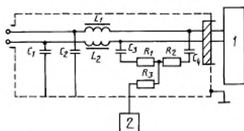
Блок связи типа М. Электрическая принципиальная схема ВЧ генератора
