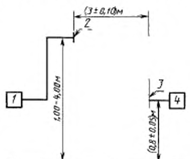
1 — ВЧ генератор; 2 — излучающая антенна; 3 — приемная антенна; 4 — измерительный приемник
