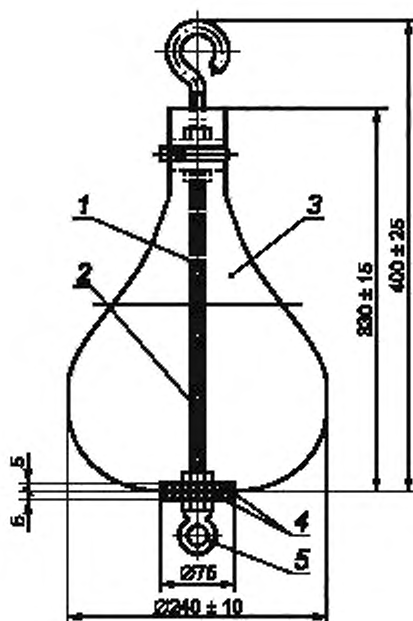
1 — стержень с нарезанной резьбой; 2 — базисная точка для измерения высоты падения в плоскости максимального диаметра, 3 — кожаный мешок; 4 — стальной диск; 5 — крепление отпускающего приспособления
