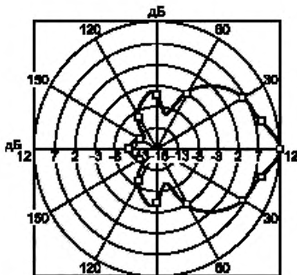
Рисунок А.5 — Диаграмма направленности D(\alpha) уровня углового распределения энергии источника для октавной полосы 1 кГц, построенная с помощью интерполяции кубическим сплайном и L_Q , рассчитанным по формуле (14)
