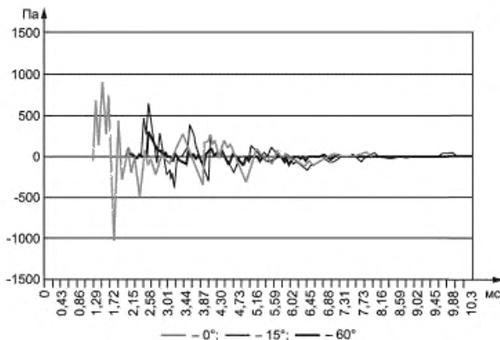
Рисунок А.1 — Зависимость звукового давления от времени для углов 0°, 15° и 60° для ствола длиной 0,67 м с полным чокм при дробовом снаряде массой 24 г с дульной скоростью 400 м/с
