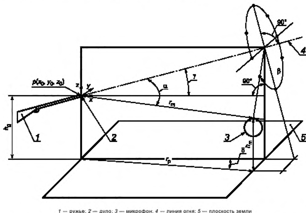
1 — ружье; 2 — дуло; 3 — микрофон; 4 — линия огня; 5 — плоскость земли
