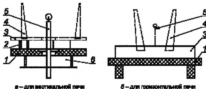
1 — огнеупорная подставка; 2 — опорные кольца; 3 — подставка с испытуемыми конусами; 4 — испытуемый конус; 5 — термопара; 6 — огнеупорная труба механического приспособления печи
