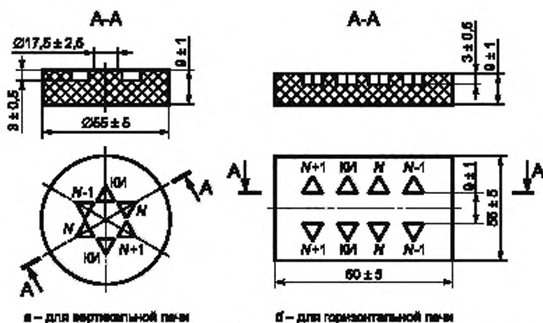
а — для вертикальной печи
