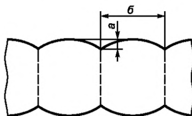
а — глубина канавок, б — ширина прилегающей панели
