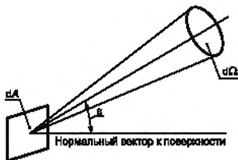
Рисунок 2 — Определение яркости
