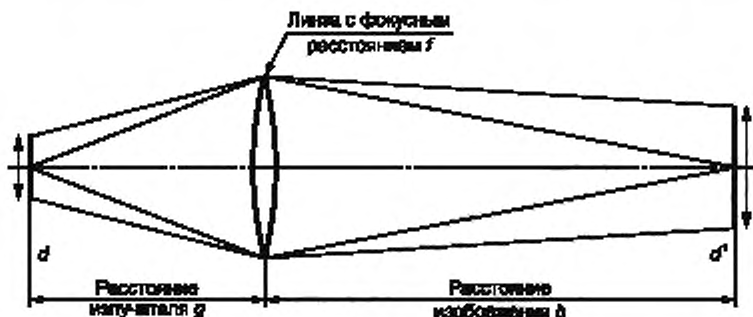
Рисунок 9 — Определение угла стягивания источника
