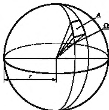
Рисунок 3 — Определение телесного угла
