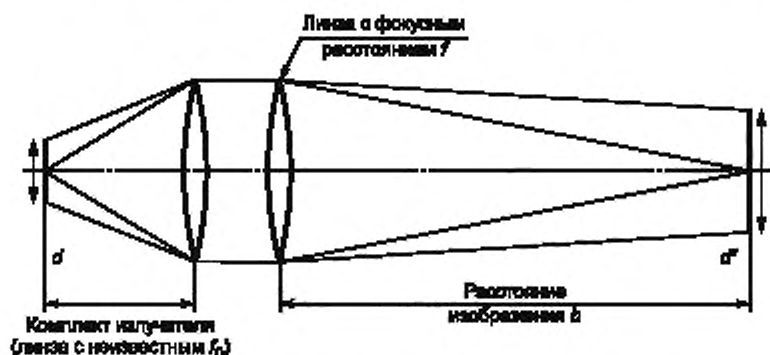
Рисунок 10 — Определение угла стягивания источника
