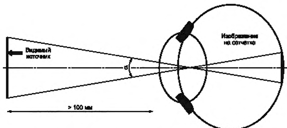
Рисунок 1 — Определение стягиваемого угла \alpha и видимого размера источника
