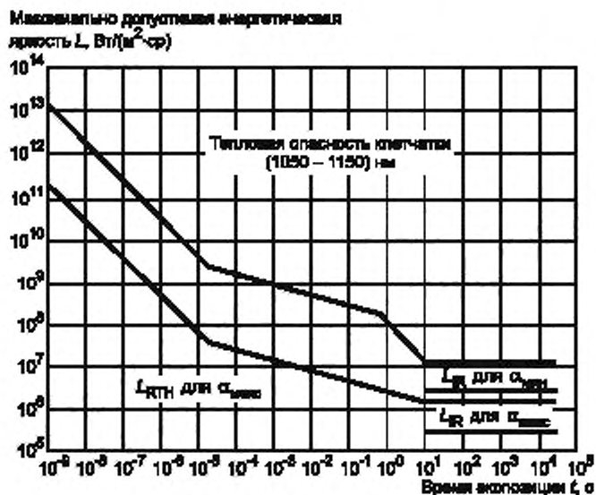
Рисунок 7 — Зависимость максимально допустимой энергетической яркости от времени при значениях L_{\text{R}} и L_{\text{RTH}}
