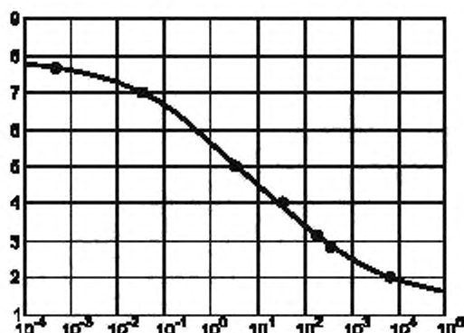
Рисунок 4 — Зависимость диаметра зрачка от яркости наблюдаемого поля в соответствии с [5].
