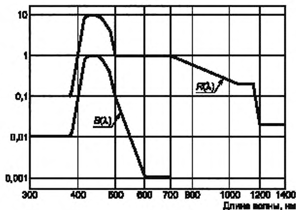
Рисунок 6 — Функция тепловой опасности клетчатки R(\lambda) и функция светлого-голубого опасения клетчатки B(\lambda)
