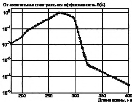
Рисунок 5 — Относительная спектральная эффективность S(\lambda)
