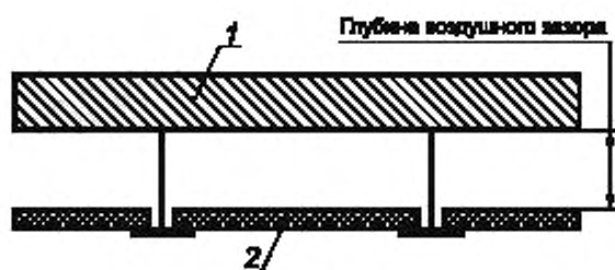
1 — поверхность помещения; 2 — звукопоглотитель
