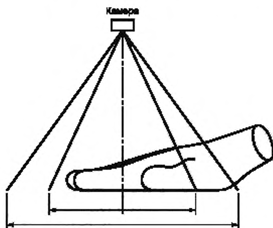
Рисунок 6 — Область интереса для измерения оптического искажения
