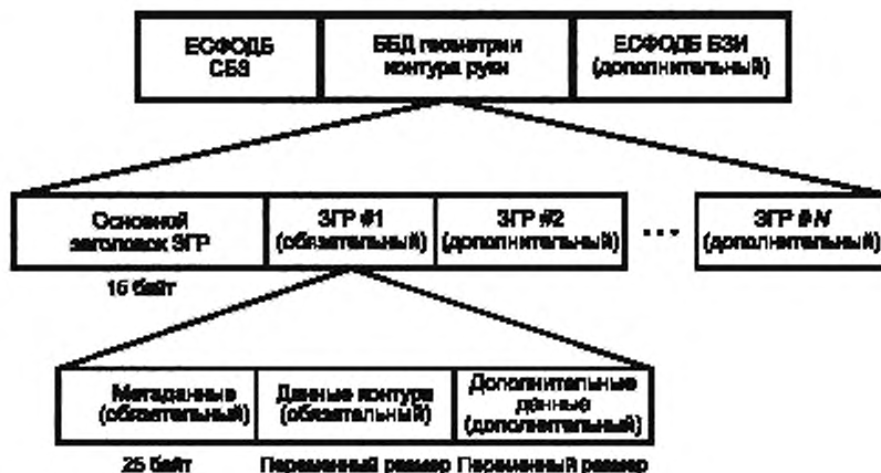
Рисунок 5 — Иерархия элементов ББД
