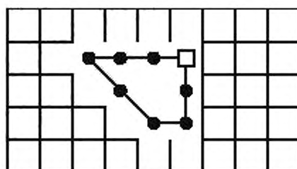
а) 8-связный ЦКФ внутренней границы = «4», «4», «4», «7», «7», «0», «2», «2»
