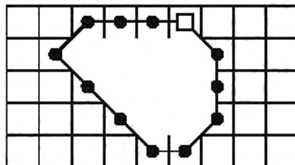
б) 8-связный ЦКФ внешней границы = «4», «4», «4», «0», «7», «7», «7», «0», «1», «2», «2», «0»
