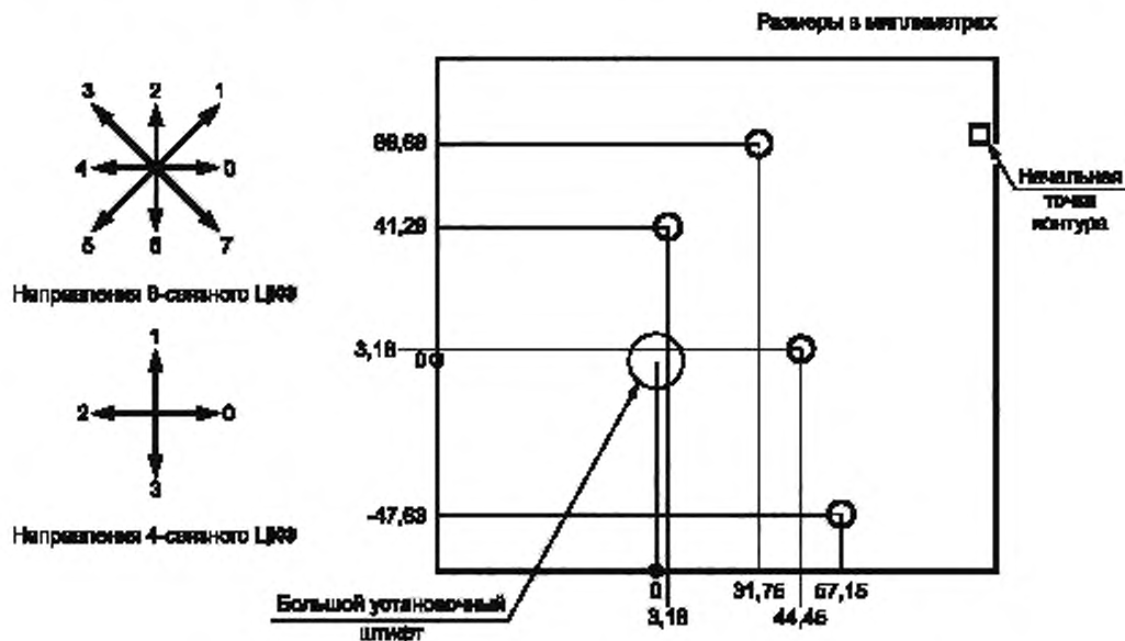
Рисунок В.1 — Примерное расположение установочных штифтов
