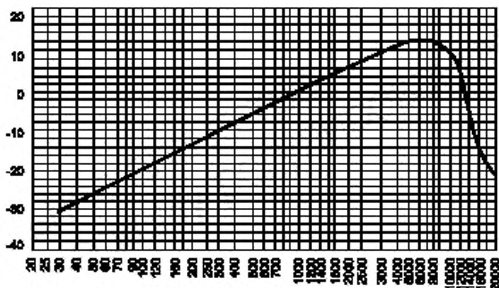
Рисунок 13 — График АЧХ псофометрического фильтра в соответствии с [4]
