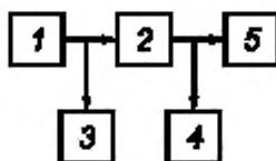
1 — низкочастотный генератор сигналов; 2 — измеряемое звено; 3 — вольтметр; 4 — измеритель нелинейных искажений или анализатор спектра; 5 — номинальное сопротивление нагрузки — резистор
