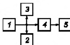
1 — низкочастотный генератор сигналов; 2 — селективный вольтметр; 3 — частотомер; 4 — канал звукового вещания; 5 — анализатор спектра или селективный вольтметр
