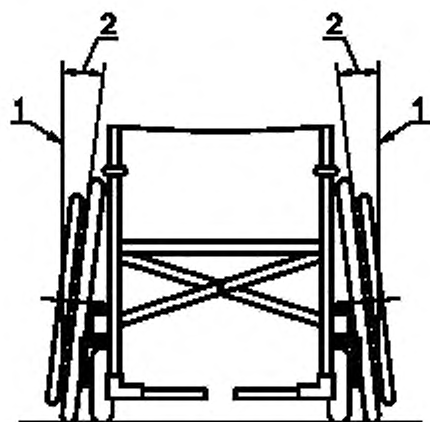
1 – вертикаль; 2 – отрицательный развал колес
