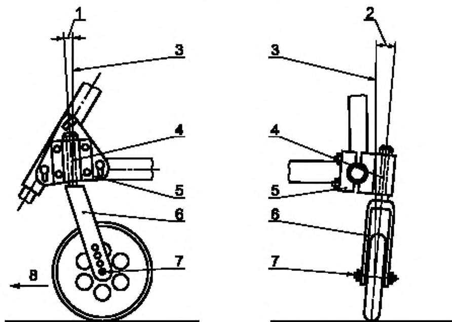
а) Узел самоориентирующегося колеса, продольная плоскость
