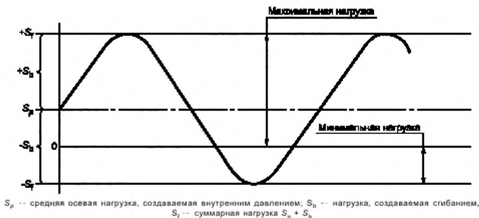
Рисунок 4 — Стандартный цикл переменной нагрузки при внутреннем давлении
