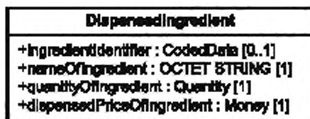
Рисунок 24 — Структура класса «DispensedIngredient»
