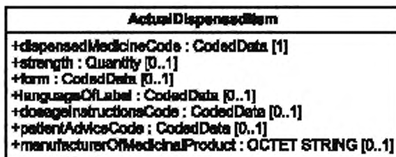
Рисунок 19 — Структура класса «ActualDispensedItem»
