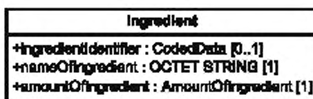
Рисунок 13 — Структура класса «Ingredient»
