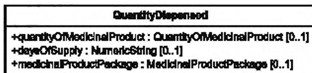
Рисунок 21 — Структура класса «QuantityDispensed»
