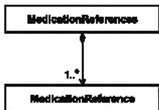
Рисунок 26 — Структура класса «MedicationReferences»
