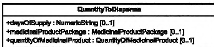
Рисунок 10 — Структура класса «QuantityToDispense»
