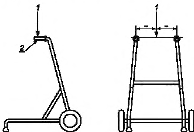
f — нагрузка; 2 — задняя контрольная точка рукоятки
