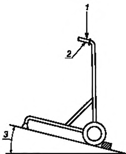
1 — нагрузка; 2 — передняя контрольная точка рукоятки, 3 — угол наклона
