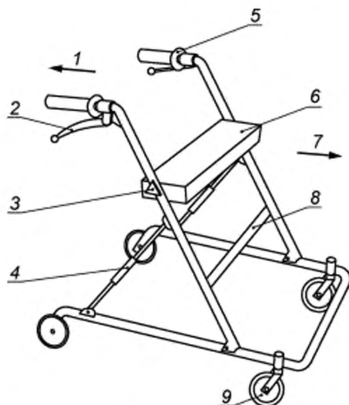
1 — направление назад; 2 — ручья тормоза; 3 — механизм регулирования высоты; 4 — механизм складывания; 5 — ручьятка/ручьа; 6 — сиденье для отдыха; 7 — направление вперед; 8 — растяжка; 9 — колесики
