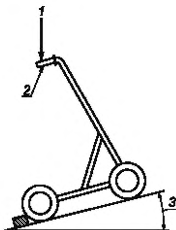
1 — нагрузка; 2 — задняя контрольная точка рукоятки; 3 — угол наклона
