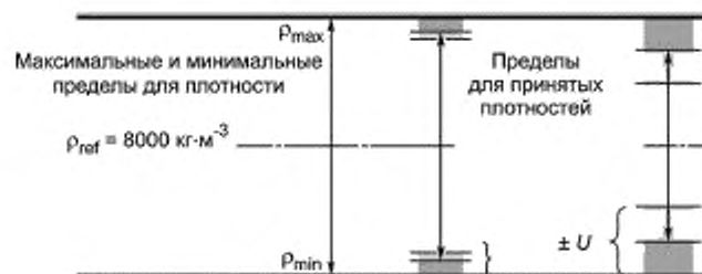
Рисунок В.3 — Допуски для плотности и пределы при проверке в зависимости от неопределенности измерений
