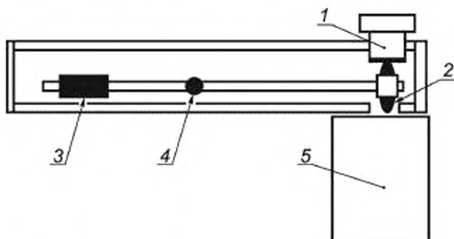
1 — стандартный образец; 2 — стержневой магнит; 3 — противовес; 4 — шарнир; 5 — гиря
