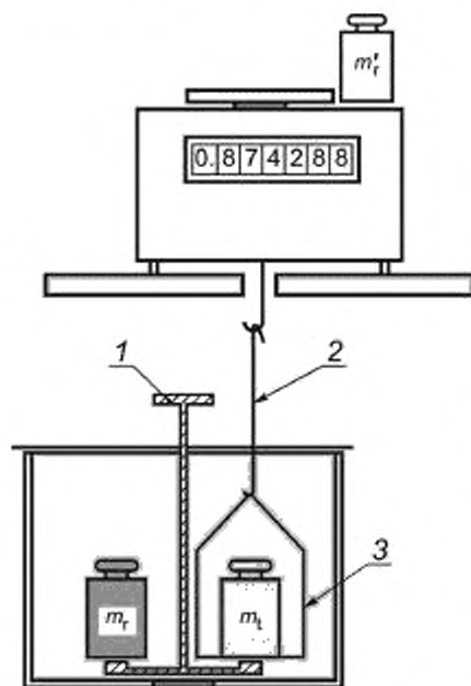
1 — устройство для смены гирь; 2 — проволочная подвеска, 3 — держатель для гири
