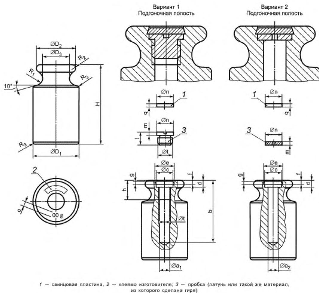
Рисунок А.1 — Примеры цилиндрических гирь
