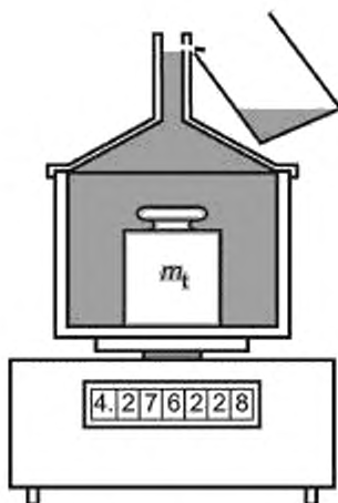
Рисунок В.7 — Иллюстрация метода D
