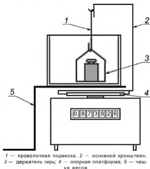
Рисунок В.5 — Иллюстрация метода В
