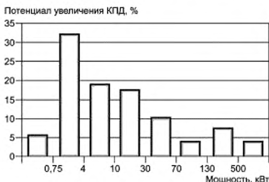
Рисунок 1 — Распределение потенциала энергосбережения двигателей по мощностям
