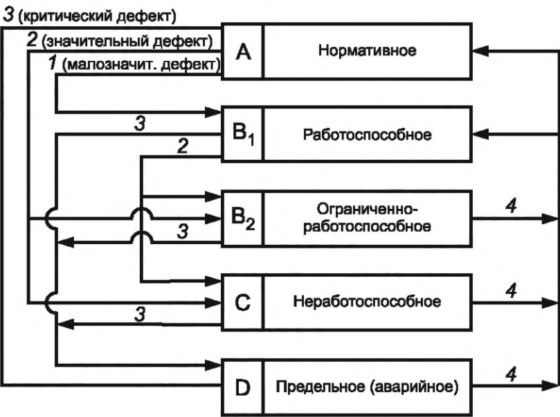
1 — отклонение отдельных характеристик технического состояния сооружения (элемента) от установленных, не приводящее к нарушению работоспособности; 2 — отказ; 3 — переход в предельное состояние из-за наличия критического дефекта; 4 — ремонт
