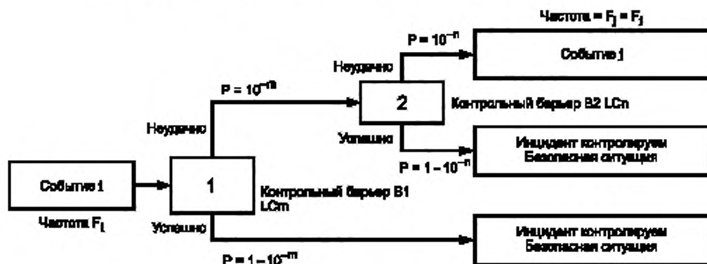
Рисунок 8 — Вероятность перехода событий с использованием барьера «Контроль»
