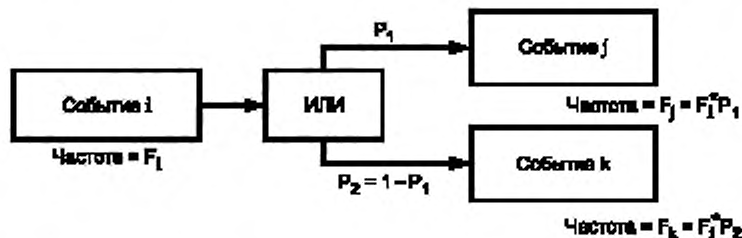
Рисунок 7 — Частота наступления каждого опасного события (ворота «ИЛИ»)
