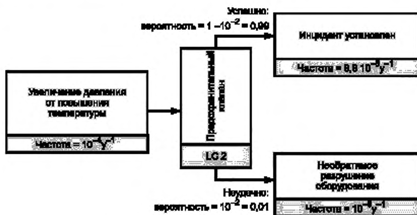
Рисунок 4 — Вероятность наступления событий в развернутом виде
