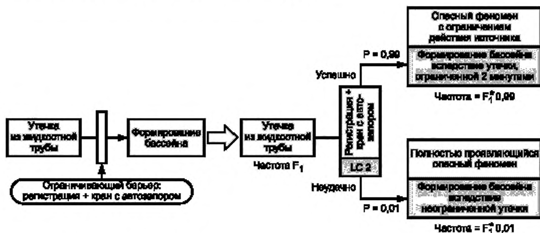
Рисунок 9 — Вероятность перехода событий с использованием барьера «Ограничение»
