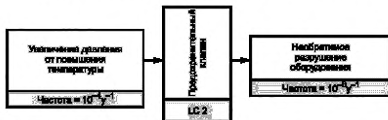
Рисунок 5 — Вероятность наступления событий в упрощенном виде
