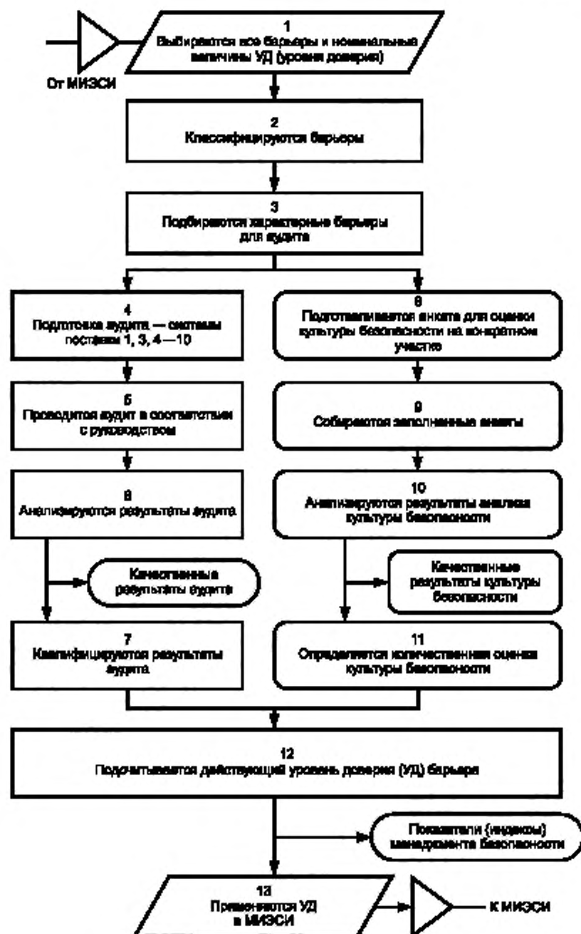
Рисунок 13 — Блок-схема оценки менеджмента безопасности
