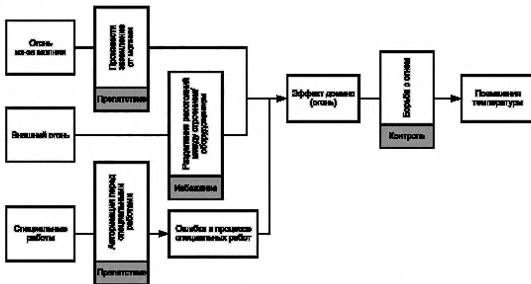
Рисунок 2 — Барьеры, размещенные на ветвях дерева отказов
