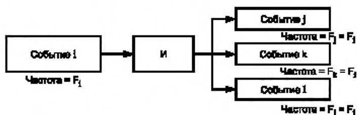
Рисунок 6 — Частота наступления каждого опасного события (ворота «И»)
