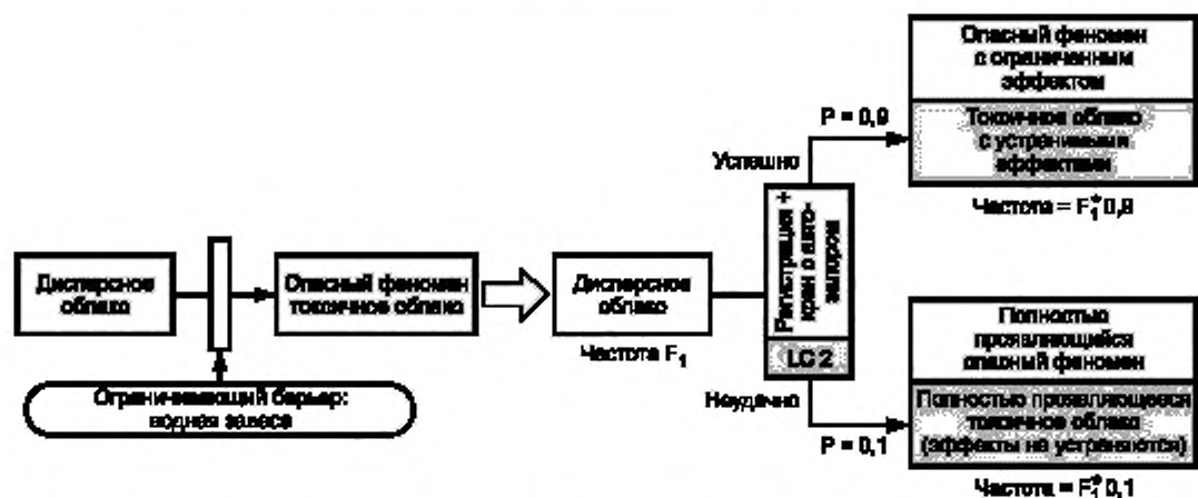
Рисунок 10 — Вероятность перехода событий с использованием барьера «Ограничение»
