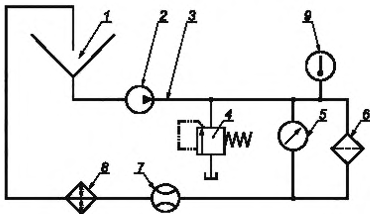
1 — введение загрязнителя; 2 — насос; 3 — другой вариант места введения загрязнителя; 4 — предохранительный клапан; 5 — дифференциальный манометр; 6 — испытываемый фильтроэлемент; 7 — расходомер; 8 — теплообменник; 9 — термометр
