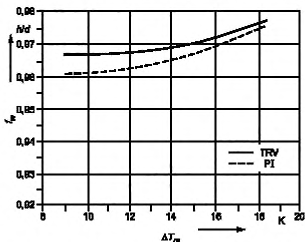
Рисунок А.1 — Коэффициент эффективности при использовании устройств контроля положения окон; старые здания ( U = 1,48 Вт/м 2 К); H — высокая масса зданий ( \sim 900 кг/м 2 )
