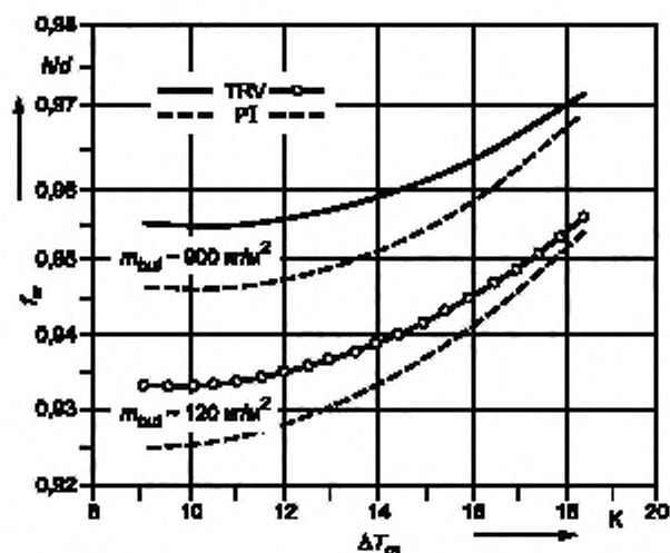
Рисунок А.2 — Коэффициент эффективности при использовании устройств контроля положения окон; новые здания ( U = 0,61 Вт/м 2 К); H — высокая масса зданий ( \sim 900 кг/м 2 ), L — низкая масса зданий ( \sim 120 кг/м 2 )
