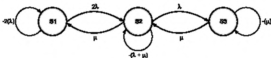
Рисунок В.10 — Пример диаграммы состояния перехода
