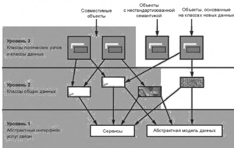
Рисунок 8 — Подход к моделированию в стандартах серии МЭК 61850
