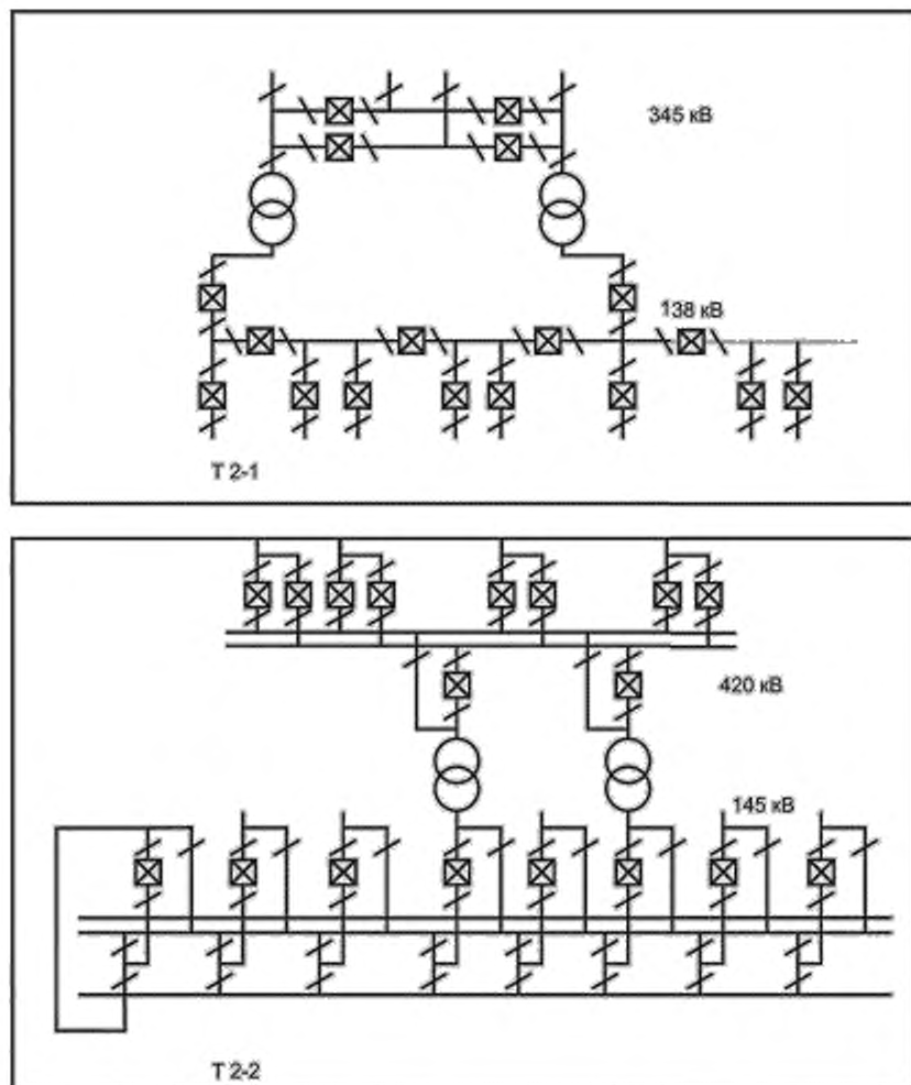
Рисунок А.5 — Пример типовых однолинейных схем подстанций типа Т 2
