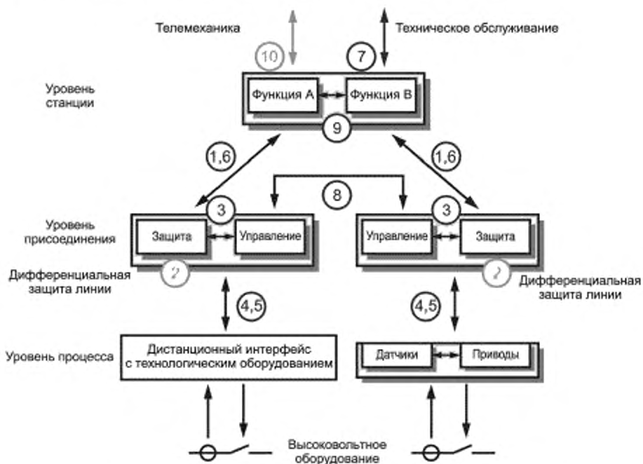
Рисунок 2 — Модель интерфейса системы автоматизации подстанции
