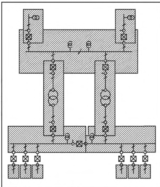
Рисунок А.8 — Типовые зоны защиты
