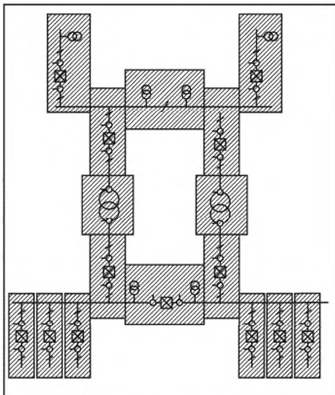
Рисунок А.7 — Деление на элементы присоединений (пример)
