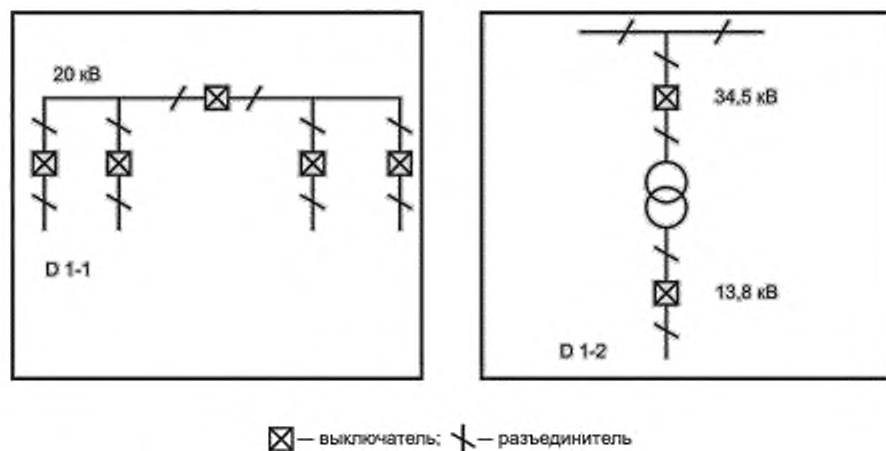
Рисунок А.1 — Примеры типовой однолинейной схемы подстанции типа D 1
