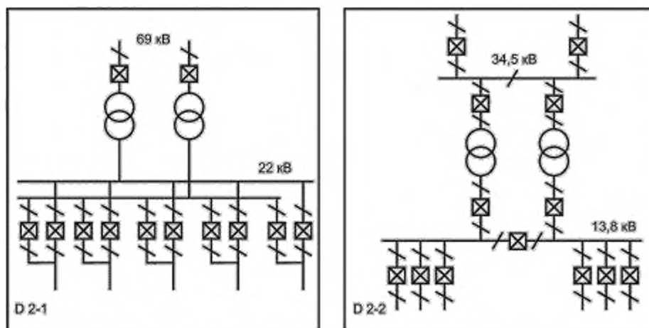
Рисунок A.2 — Примеры типовых однолинейных схем подстанций типа D 2
