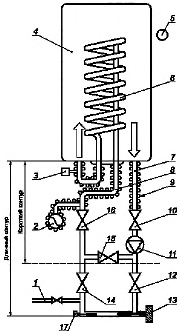
1 — подпиточная труба; 2 — изолированный расширительный бак; 3 — расширительный клапан; 4 — испытуемый резервуар; 5 — внешний термометр; 6 — нагревающий змеевик; 7 — точка измерения температуры T_1 ; 8 — точка измерения температуры T_2 ; 9 — теплоизоляция; 10, 12, 14, 15, 16 — клапаны; 11 — циркуляционный насос; 13 — электронагреватель; 17 — термостат
