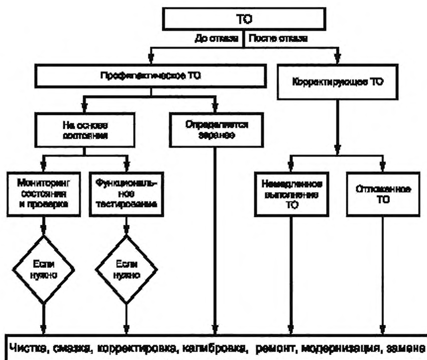
Рисунок 2 — Типы работ по техническому обслуживанию
