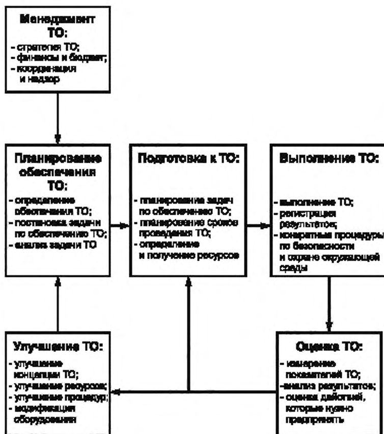
Рисунок 3 — Процессы технического обслуживания
