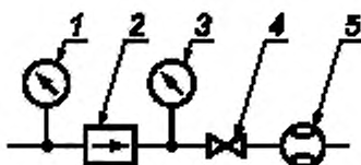
1 — манометр для измерения давления P_1 на входе (класс точности не ниже I); 2 — испытываемое устройство; 3 — манометр для измерения давления P_2 на выходе (класс точности не ниже I); 4 — вентиль; 5 — расходомер
