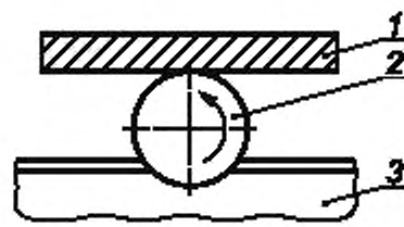
1 — образец, 2 — валик; 3 — битум
