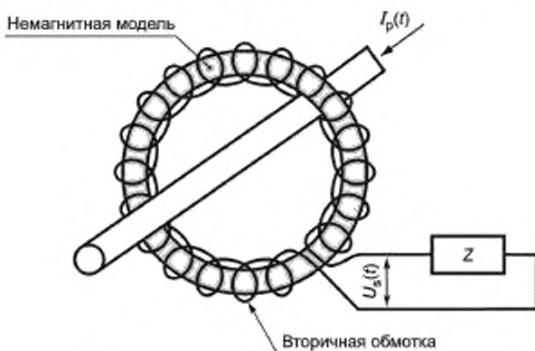
Рисунок С.4 — Автономная катушка без сердечника
