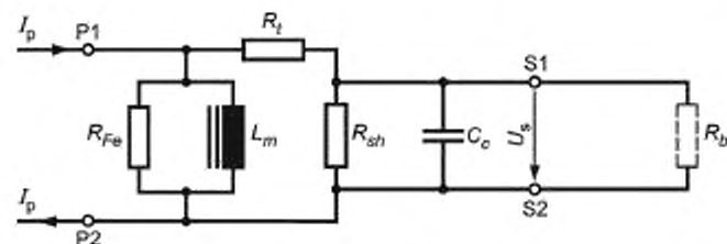
Рисунок С.2 — Трансформатор с ферродинамическим сердечником
