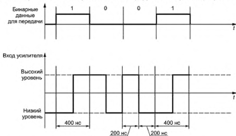
Рисунок 4 — Манчестерское кодирование
