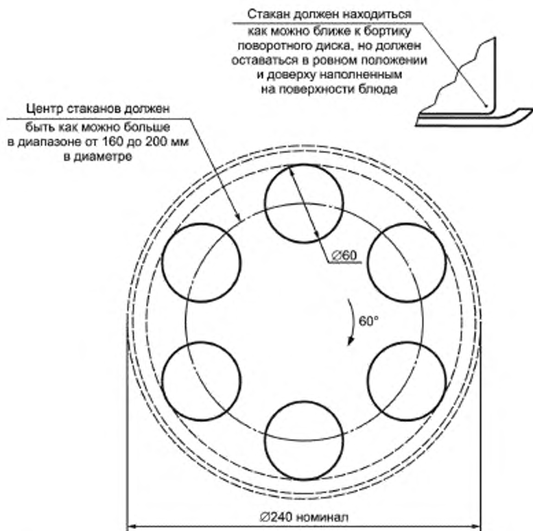
Рисунок 1 — Расположение стаканов на поворотном диске микроволновой печи
