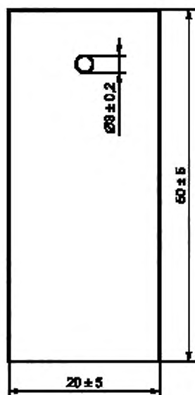
Рисунок 2 — Образец (пластина)
