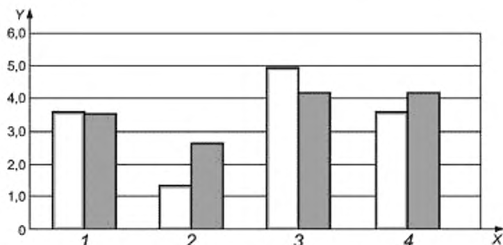
Рисунок Е.1 — Диаграмма сравнения измеренного и вычисленного ожидаемого содержания загрязняющего вещества при допущении, что при равномерном введении индикаторного газа может быть получена информация о распределении источников загрязняющего вещества
