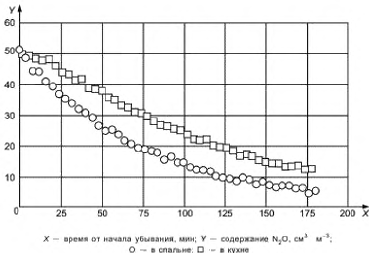
Рисунок D.1 — График зависимости содержания индикаторного газа от времени
