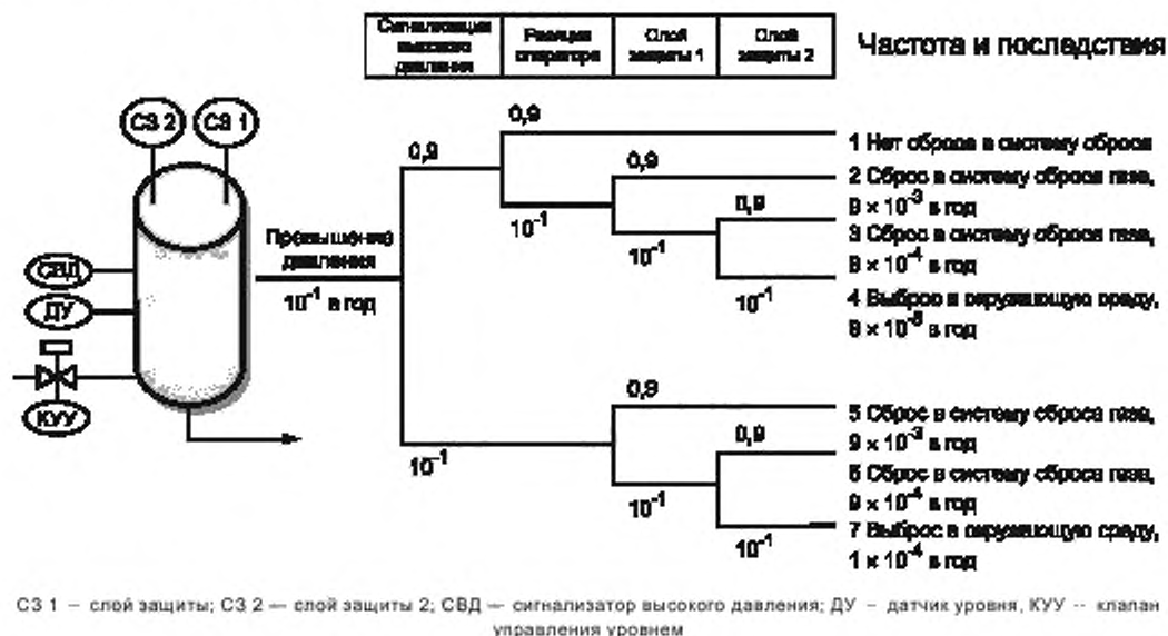
Рисунок В.4 — Опасные события при резервированном слое защиты
