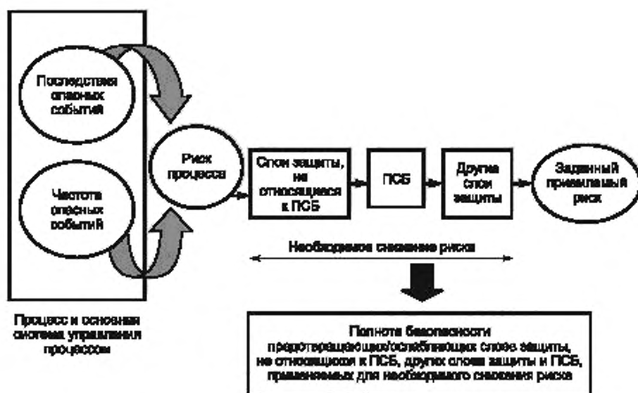
Рисунок 4 — Концепция риска и полноты безопасности
