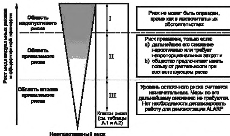
Рисунок А.1 — Приемлемый риск и принцип ALARP
