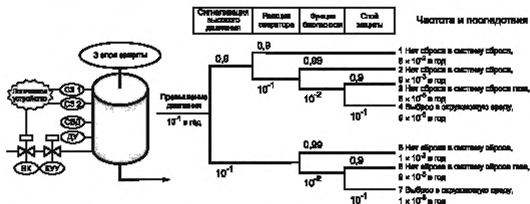
Рисунок В.5 — Опасные события при функции безопасности ПСБ с УПБ 2
