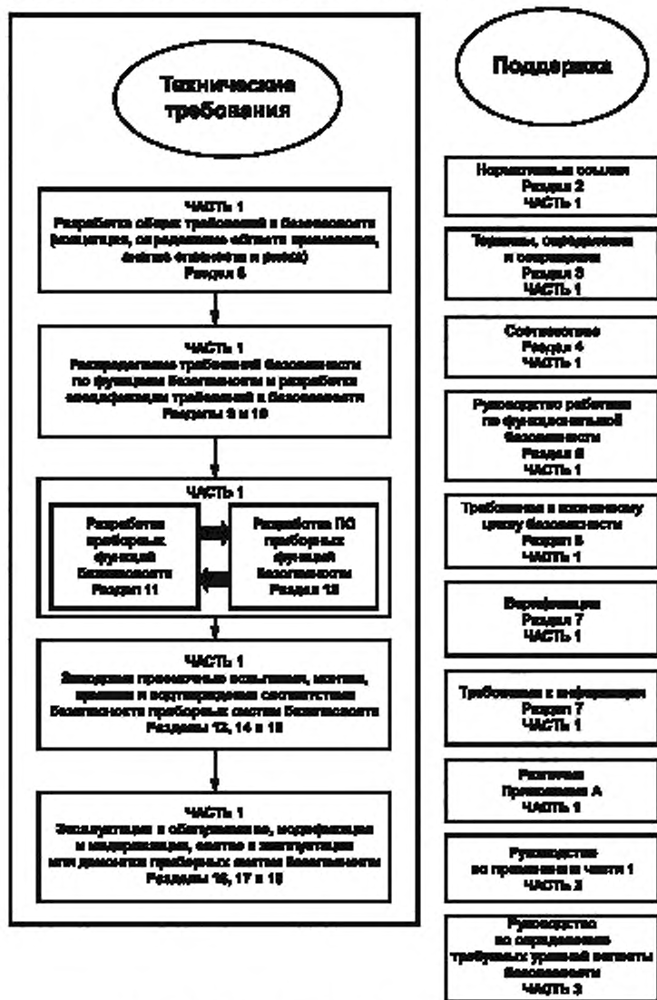
Рисунок 1 — Общая структура настоящего стандарта
