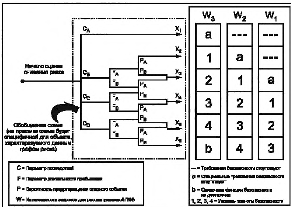
Рисунок D.1 — Граф риска, общая схема
