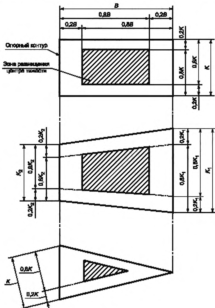
Рисунок 1 — Конфигурация основания грузоподъемного крана
