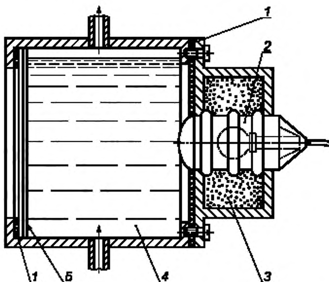
Рисунок 1 — Рекомендуемое устройство для испытания светильников, передняя часть которых соприкасается с водой
