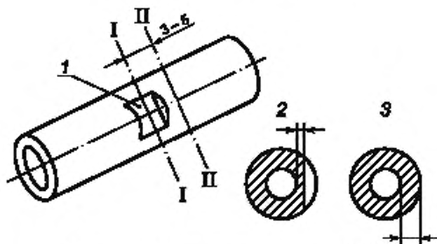
1 — отпечаток; 2 — сечение I—I; 3 — сечение II-II
