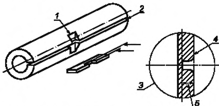
1 — отпечаток; 2 — вырезанная тонкая полоска; 3 — вид вырезанной полоски под микроскопом; 4 — перекрестие микроскопа; 5 — глубина отпечатка
