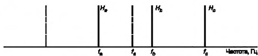
Рисунок G.1 — Примеры выбора частоты H_c
