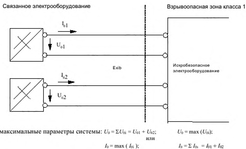
Рисунок В.3 – Последовательные и параллельные соединения. Суммирование значений напряжения и тока
