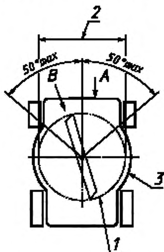
1 — траектория лезвия; 2 — ширина лезвия; 3 — ограждение лезвия
