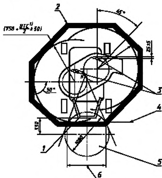
Рисунок ВВ.3 — Многошпindleная косилка. Испытательное ограждение
