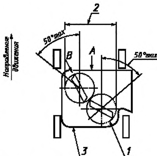
1 — траектория лезвия; 2 — ширина лезвия; 3 — ограждение лезвия
