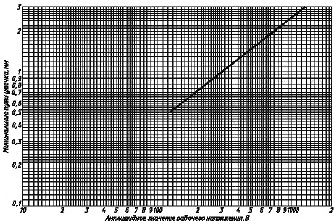
Рисунок 1 — Пути утечки между проводниками на печатных платах, не предназначенными для присоединения к сети
