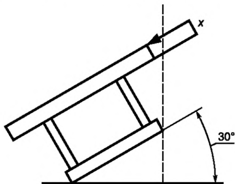
Рисунок 7 — Сиденье-колыбель
