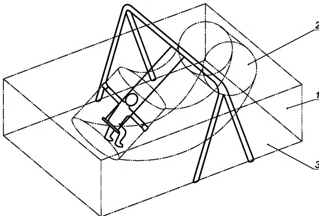
Рисунок 9 — Зоны качелей
