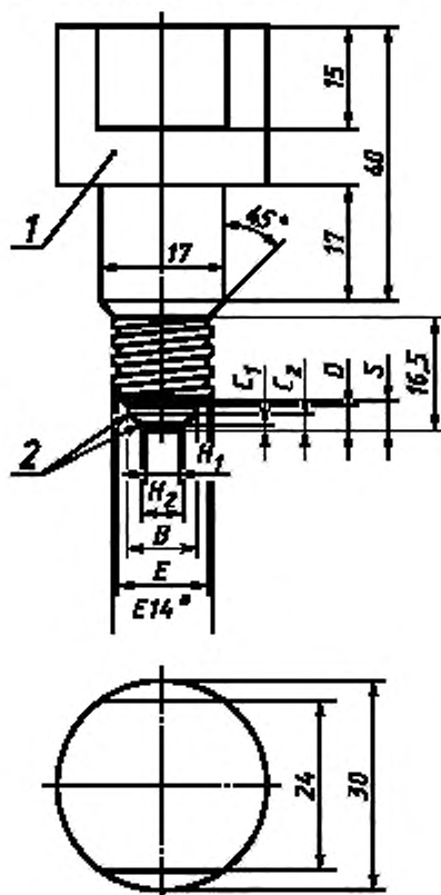
Испытательный цоколь А
