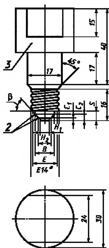
Испытательный цоколь В
