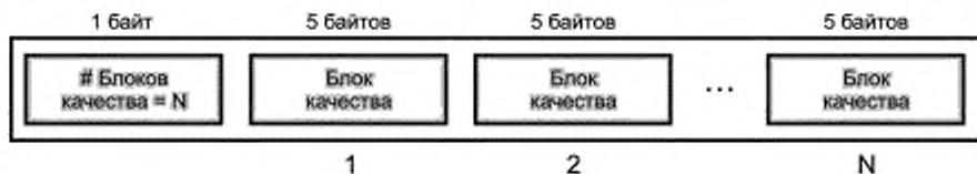
Рисунок 3 — Структура поля качества
