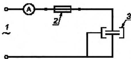
1 — источник переменного напряжения; 2 — плавкий предохранитель; 3 — конденсатор
