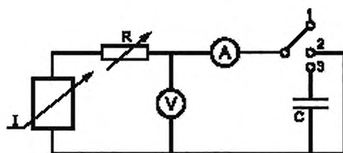
Рисунок 2 — Схема выдержки на постоянном напряжении
