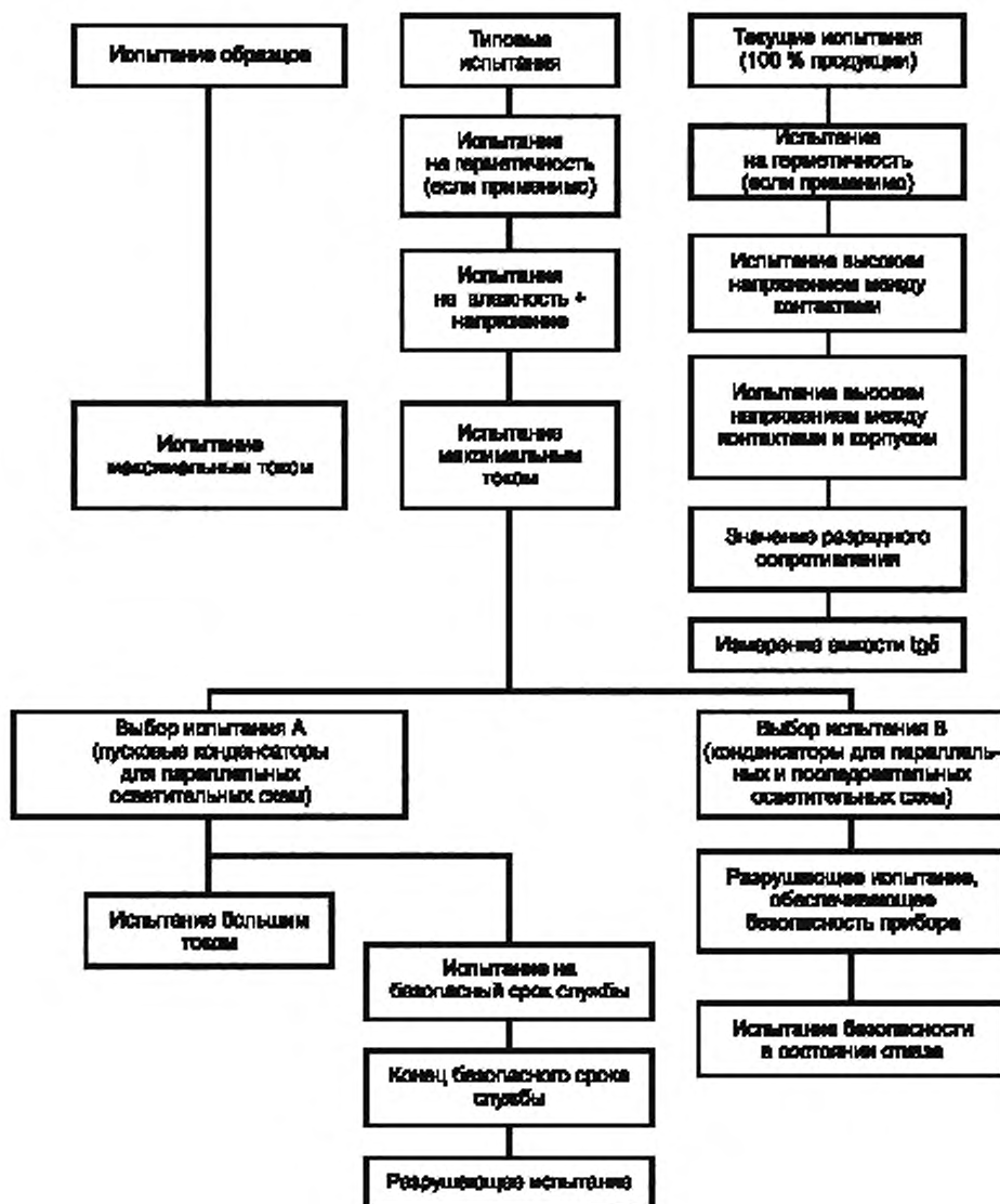
Рисунок 4 — Схема процедуры испытаний
