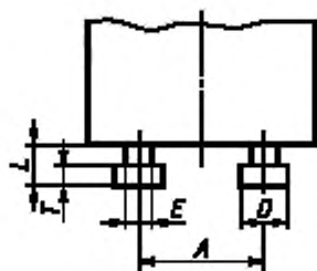
Рисунок 21 — Стартер для испытания по разделу 13
