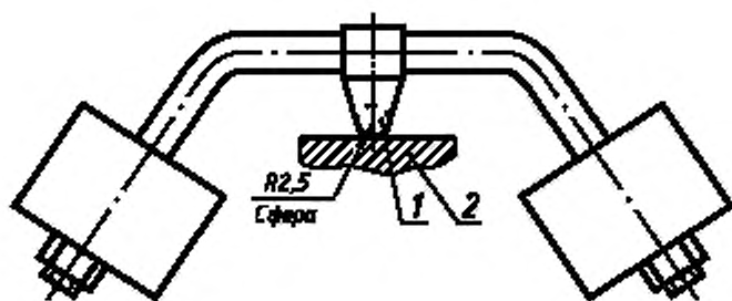
Рисунок 7 — Устройство для вдавливания шарика
