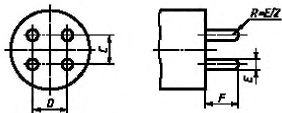
Рисунок 19 — Испытательный цоколь для испытания патронов G10q по разделу 13
