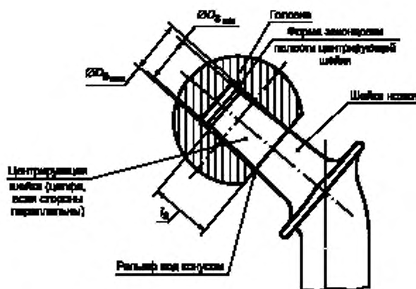
Рисунок 2 — Головка, закрепленная на центрирующей шейке или цапфе (головка альтернативной конструкции)
