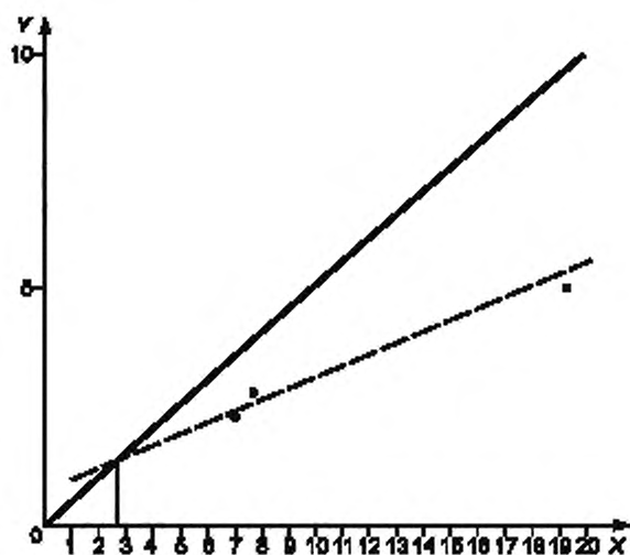
X — содержание хрома в межлабораторных тестах (2003—2005 гг.) Y — отклонения от среднего содержания
