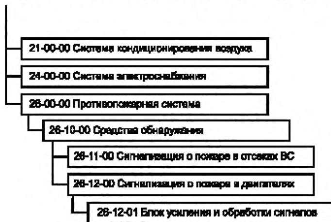
Рисунок 2 — Использование СНК для идентификации СЧ ВС
