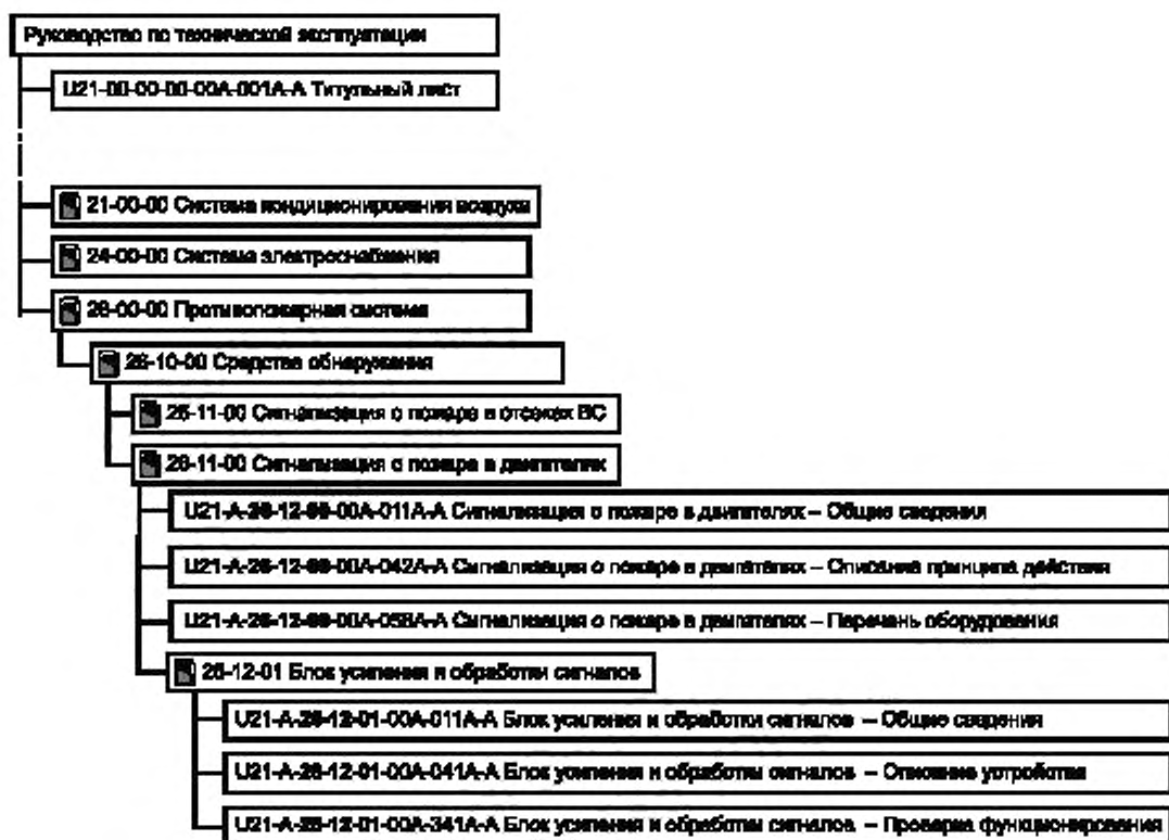
Рисунок 3 — Использование СНК для идентификации структурных элементов ЭД
