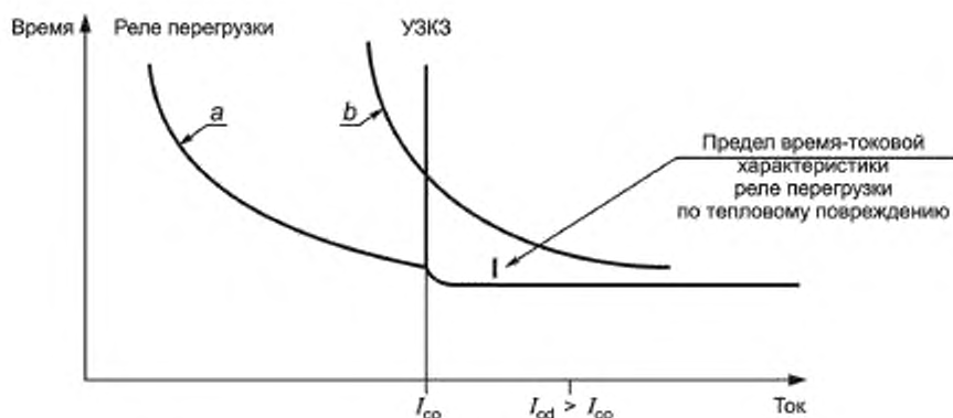
Рисунок В.1б — Координация с автоматическим выключателем
