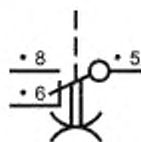
Переключающий контакт с замедлением в обоих направлениях
