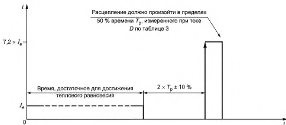
Рисунок 8 — Испытание тепловой памяти
