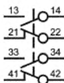
Четыре контактных элемента
