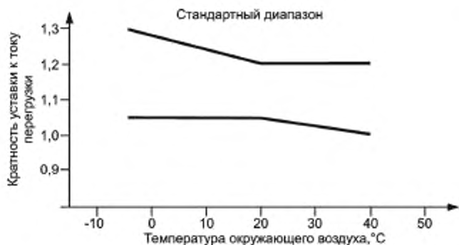
Рисунок 7 — Зависимости пределов кратности уставок тока от температуры окружающего воздуха для компенсированных реле перегрузки с выдержкой времени (см. 8.2.1.5.1)
