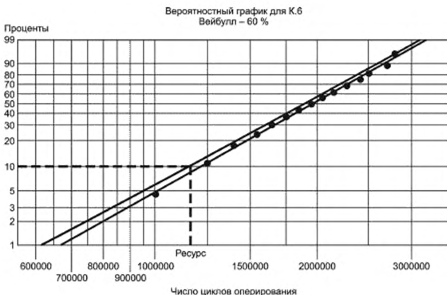
Рисунок К.1 — График медианной ранговой регрессии
