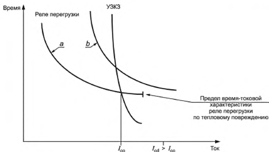
Рисунок В.1а — Координация с плавким предохранителем
