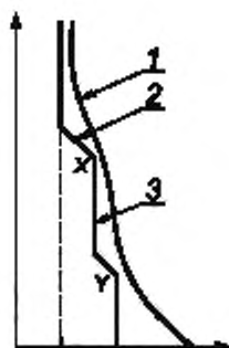
1 — преддугговая характеристика; 2 — прямая постоянного значения I^2t ; 3 — условная кривая перегрузок
