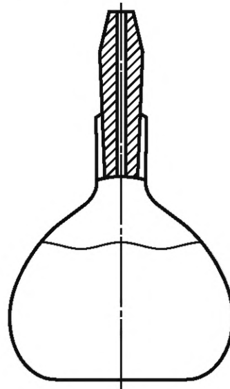
Рисунок 2 — Стеклоанный пикнометр типа Гей-Люссака
