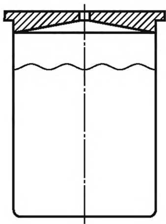
Рисунок 1 — Металлический пикнометр
